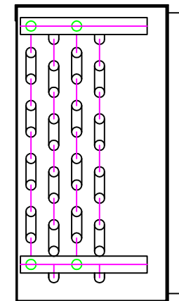
左视图 HEADER END
